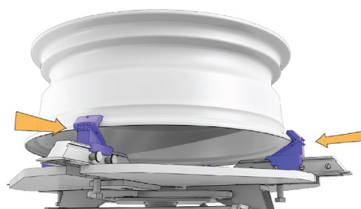
Serrage externe
